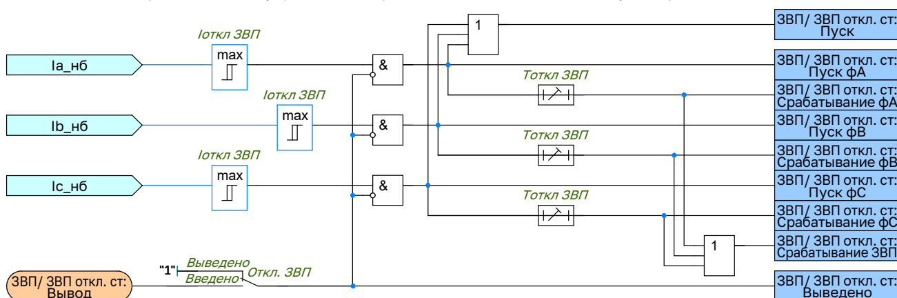
Рисунок 2.10 – Функциональная схема логики ступеней ЗВП
