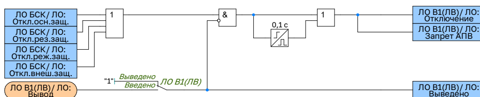
Рисунок 2.34 – Функциональная схема логики отключения В1(ЛВ)ВН
